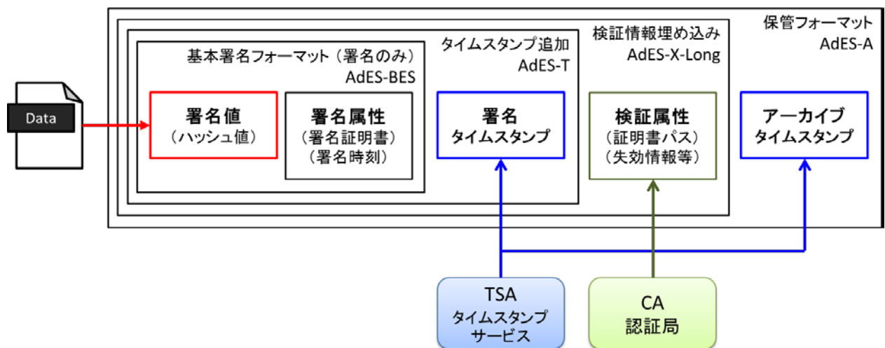
図 10 長期署名フォーマットの構造
